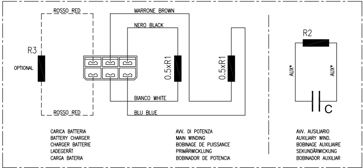
STATOR - STATOR - STATOR - STATOR - ESTATOR
