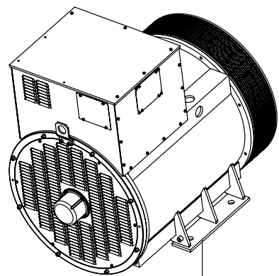
ERDUNGSANSCHLUSS
